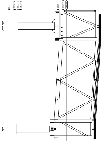
CORTE CC Esc. 1/10
