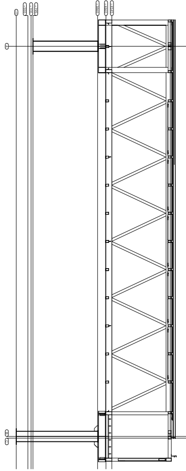
CORTE AA Esc. 1/10
