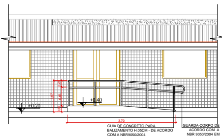
VISTA EXTERNA DA RAMPA ESCALA 1:50
