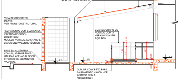
CORTE PARCIAL 01 ESCALA 1:50
