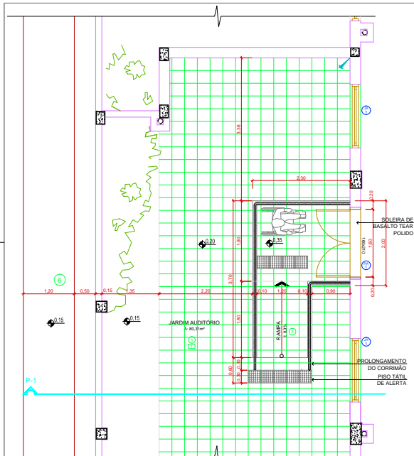
PLANTA BAIXA - JARDIM AUDITÓRIO ESCALA 1:50
