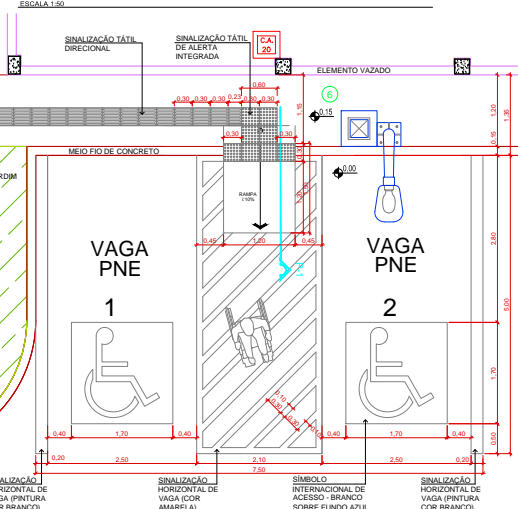
PLANTA BAIXA ESCALA 1:50
