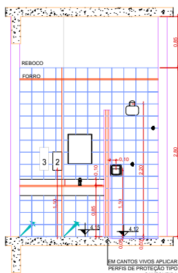
ELEVACÃO 01 ESCALA 1:20
