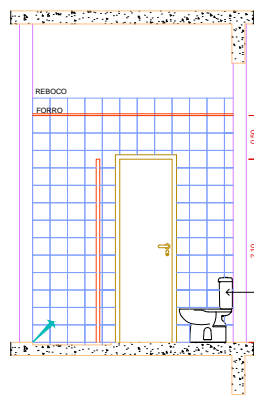
ELEVACÃO 03 ESCALA 1:20
