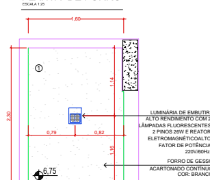
PLANTA DE FORRO ESCALA 1:20
