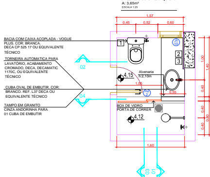
PLANTA BAIXA A: 3,65m² ESCALA 1:20
