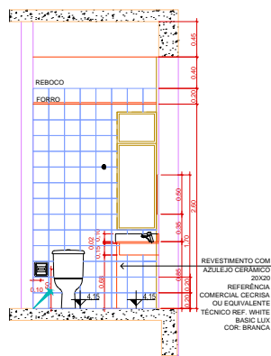
ELEVACÃO 02 ESCALA 1:20
