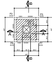
FORMA DA TAMPA NÍVEL +825
