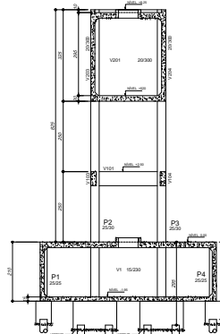
Corte A-A
