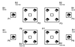
FORMA DE FUNDAÇÃO
