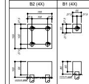
DETALHE DOS BLOCOS
