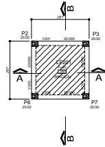
FORMA DO FUNDO NÍVEL +520
