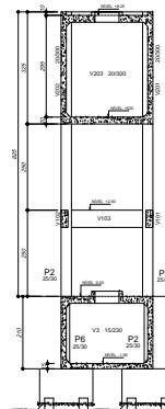
Corte B-B
