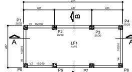
FORMA DO FUNDO DA CISTERNA (NÍVEL -1,95)
