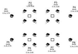
PLANTA DE ESTAQUEAMENTO
