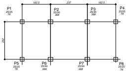
PLANTA DE LOCAÇÃO E PLANTA DE CARGAS
