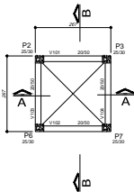
FORMA DO NÍVEL +250
