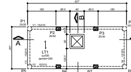
FORMA DA TAMPA DA CISTERNA (NÍVEL 0,00)
