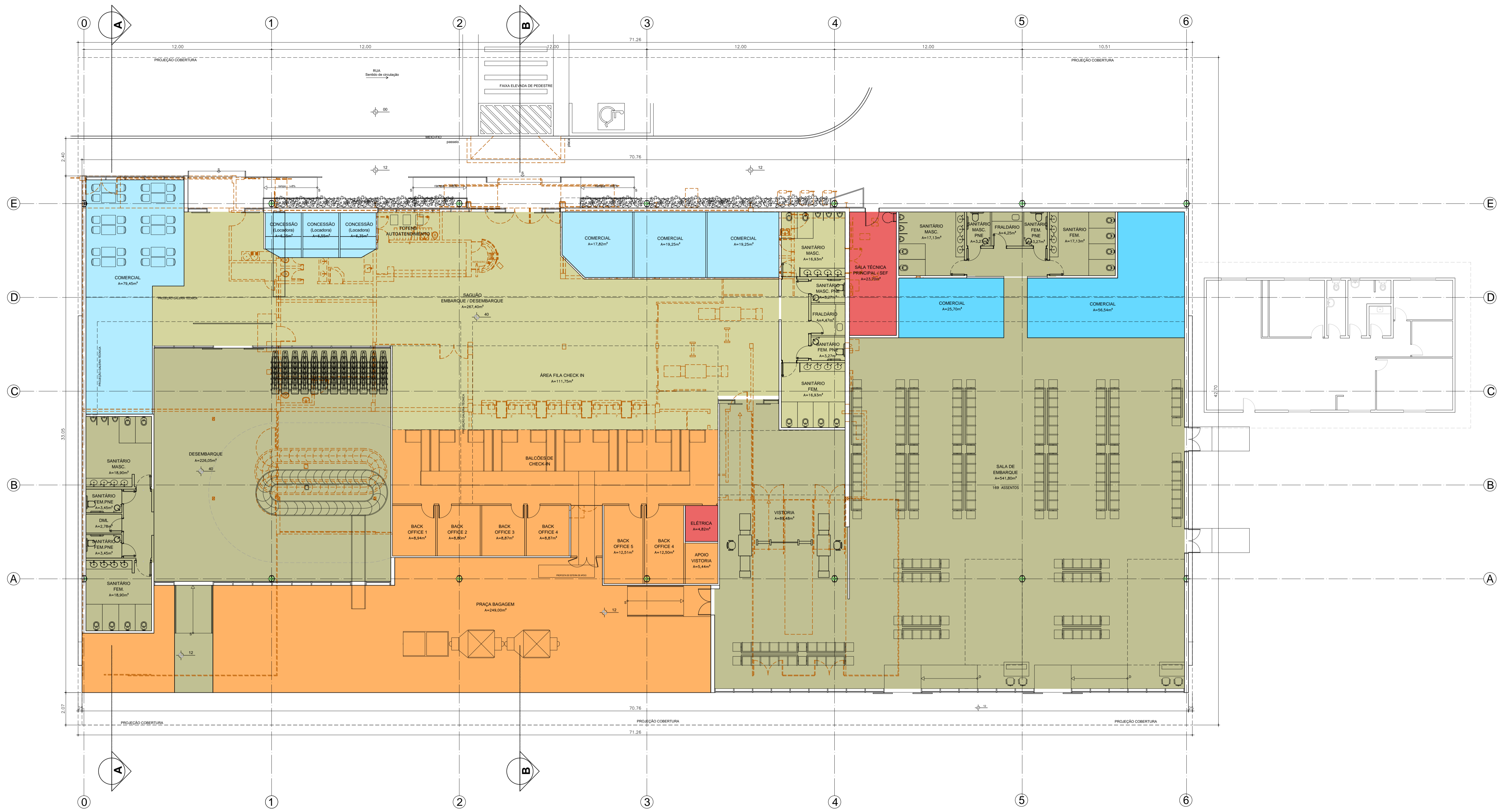
PLANTA BAIXA - TÉRREO PROPOSTA ESC. 1/125
