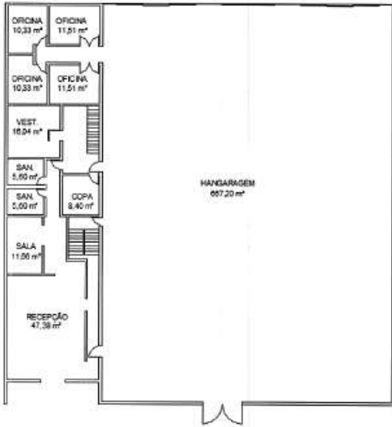
Planta Baixa Térreo
