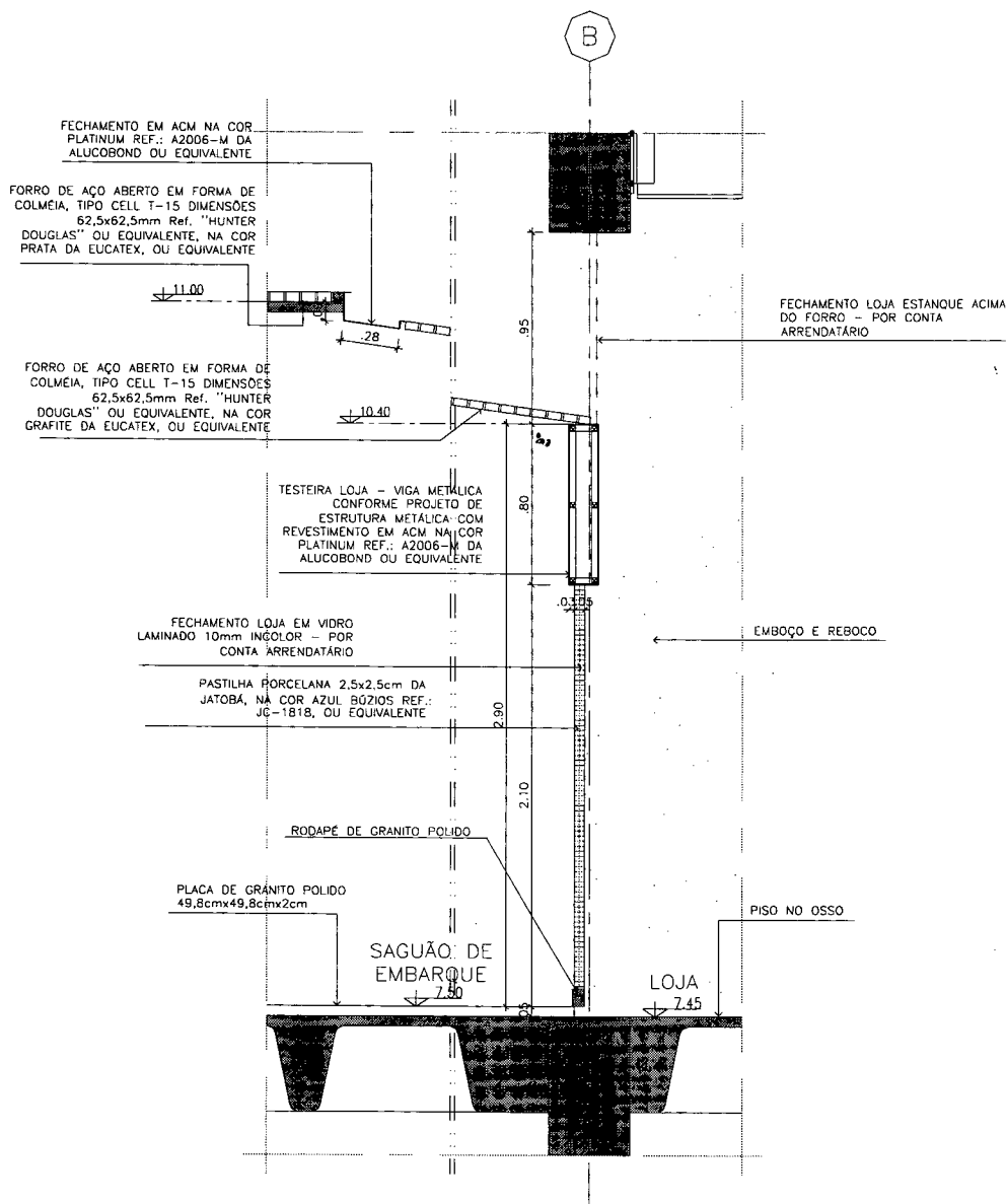
DETALHE 18 LOJAS EIXO "B - 06 E 12" - 1º PAVIMENTO (NÍVEL 7.50)
