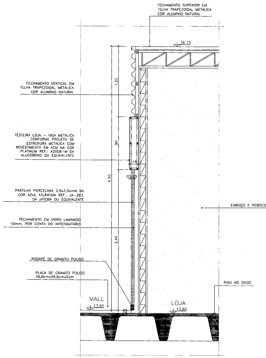
DETALHE 19 LOJAS - 2º PAVIMENTO (NÍVEL 13.65)
