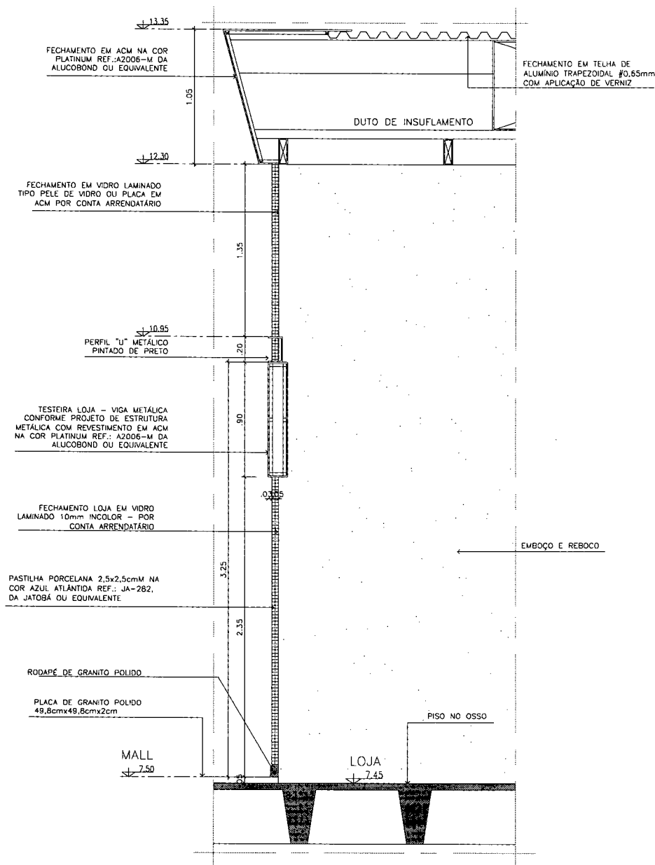
DETALHE 17 LOJAS EIXO "F" / 01 A 06 - 12 A 17" - 1º PAVIMENTO (NÍVEL 7.50)
