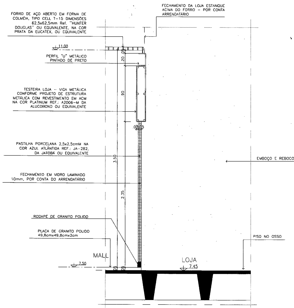
DETALHE 12 LOJAS EIXO "F" / 06 A 12" - 1º PAVIMENTO (NÍVEL 7.50)
