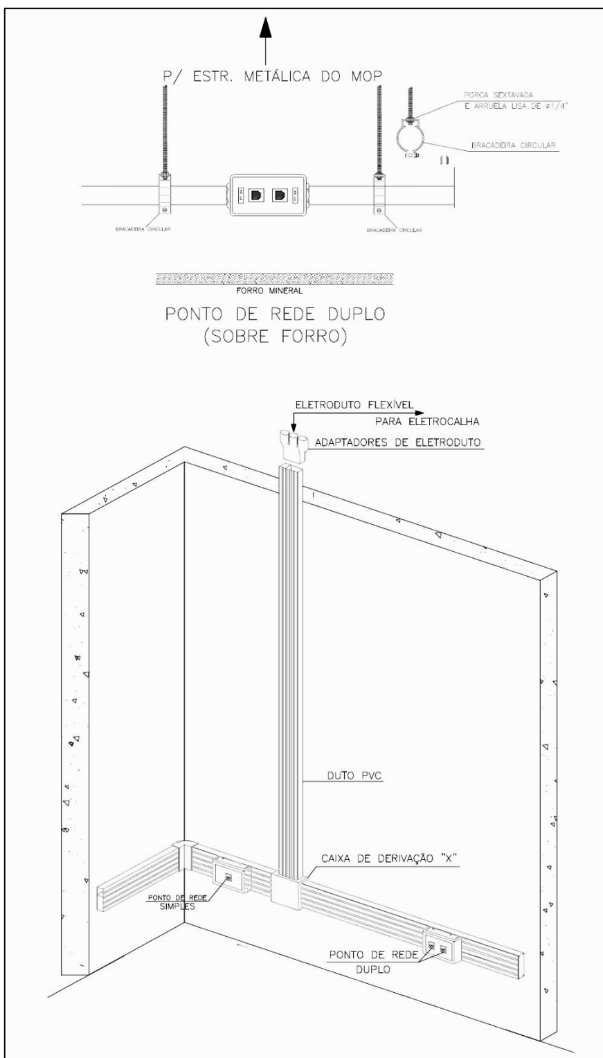
DETALHES PONTOS DE REDE
