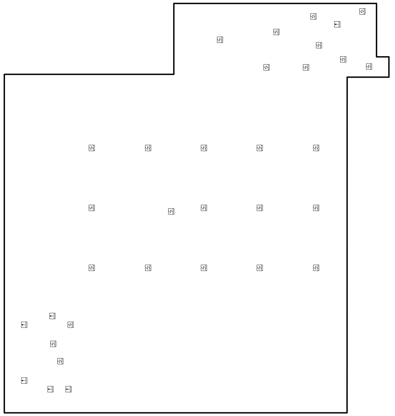
PLANTA BAIXA FORNO PAVIMENTO SUPERIOR - SISTEMA DE DETECCAO ESCALA 1:500
