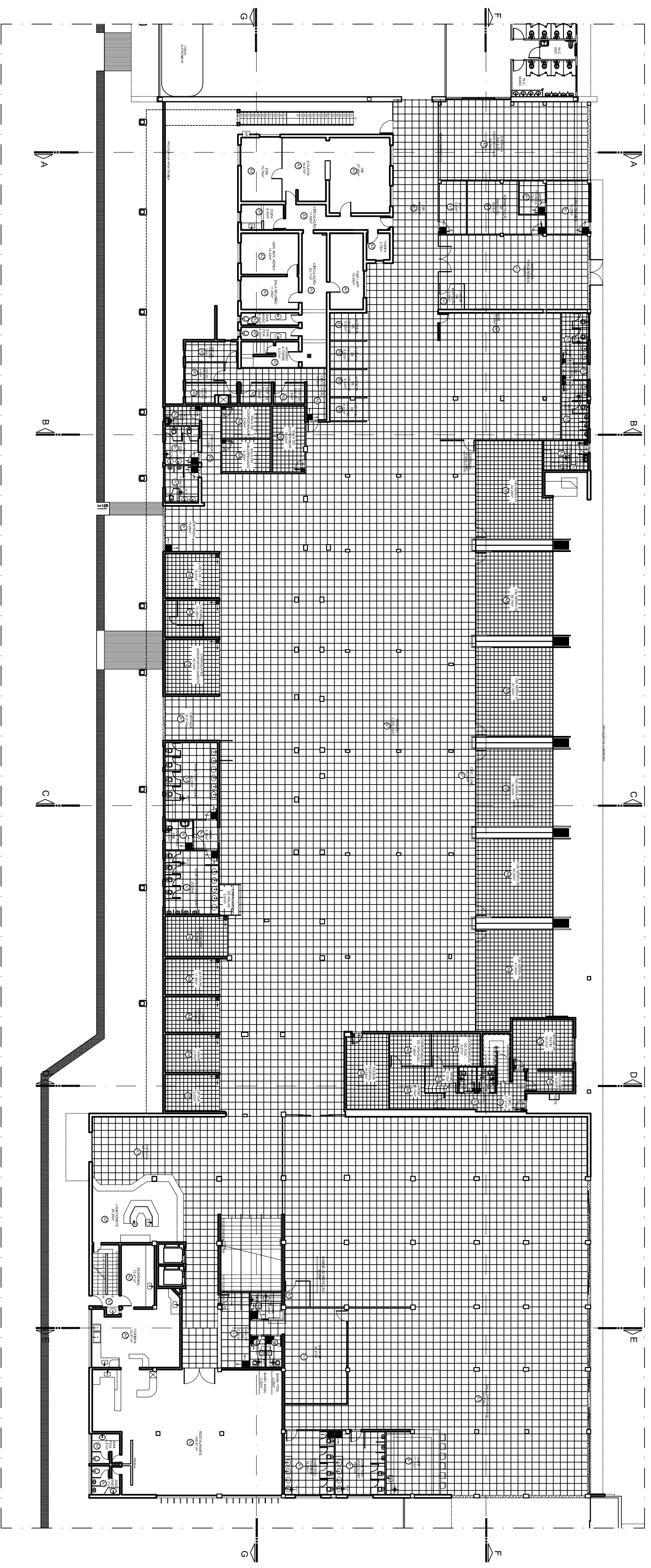
PLANTA BAWA - PAV. TERREO DESEMBANQUE/AGUIAR/BAUQUE PAG. DE PISO ESCALA 1:150
