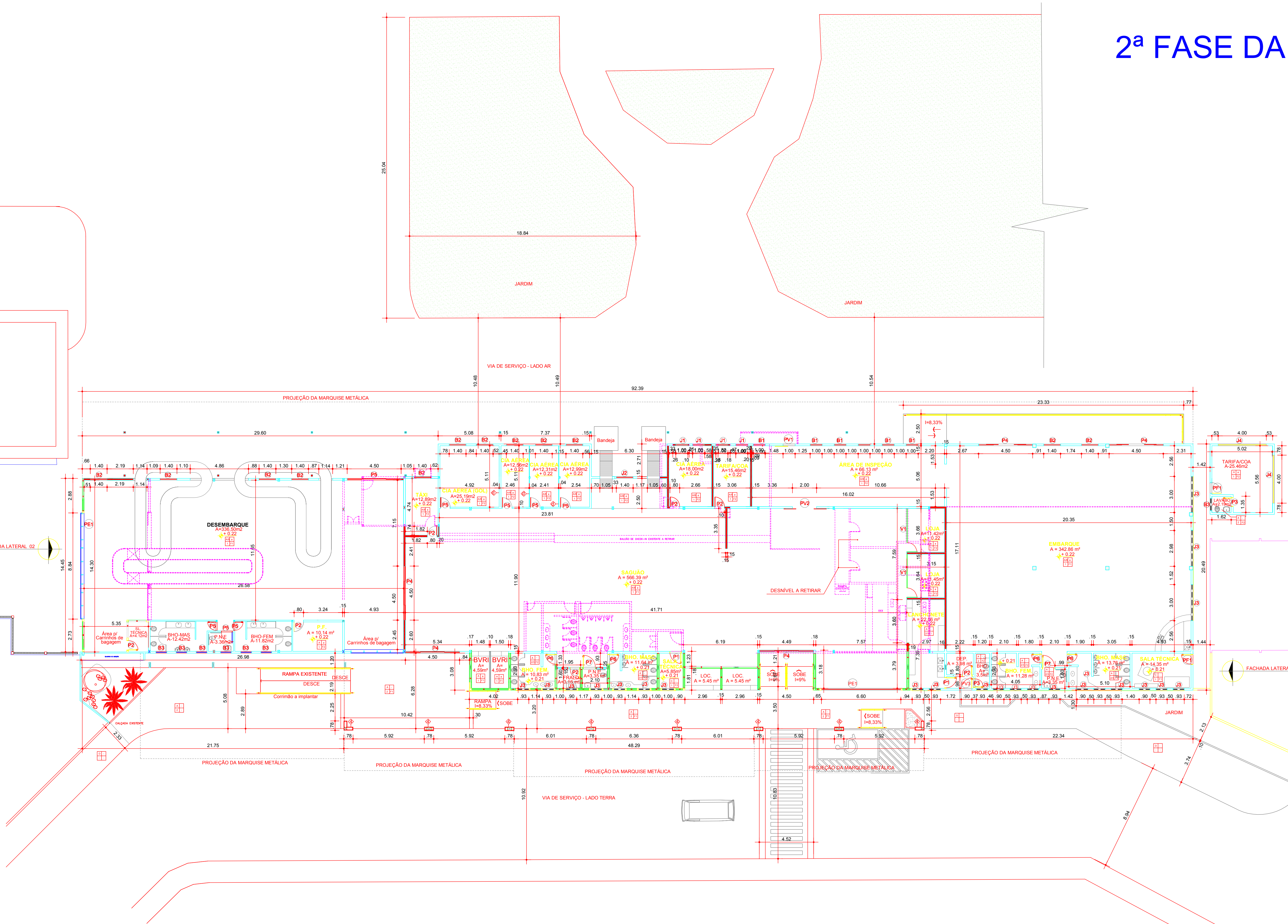
PLANTA DE DEMOLIÇÕES - 2ª FASE DA OBRA - TPS MARABÁ
