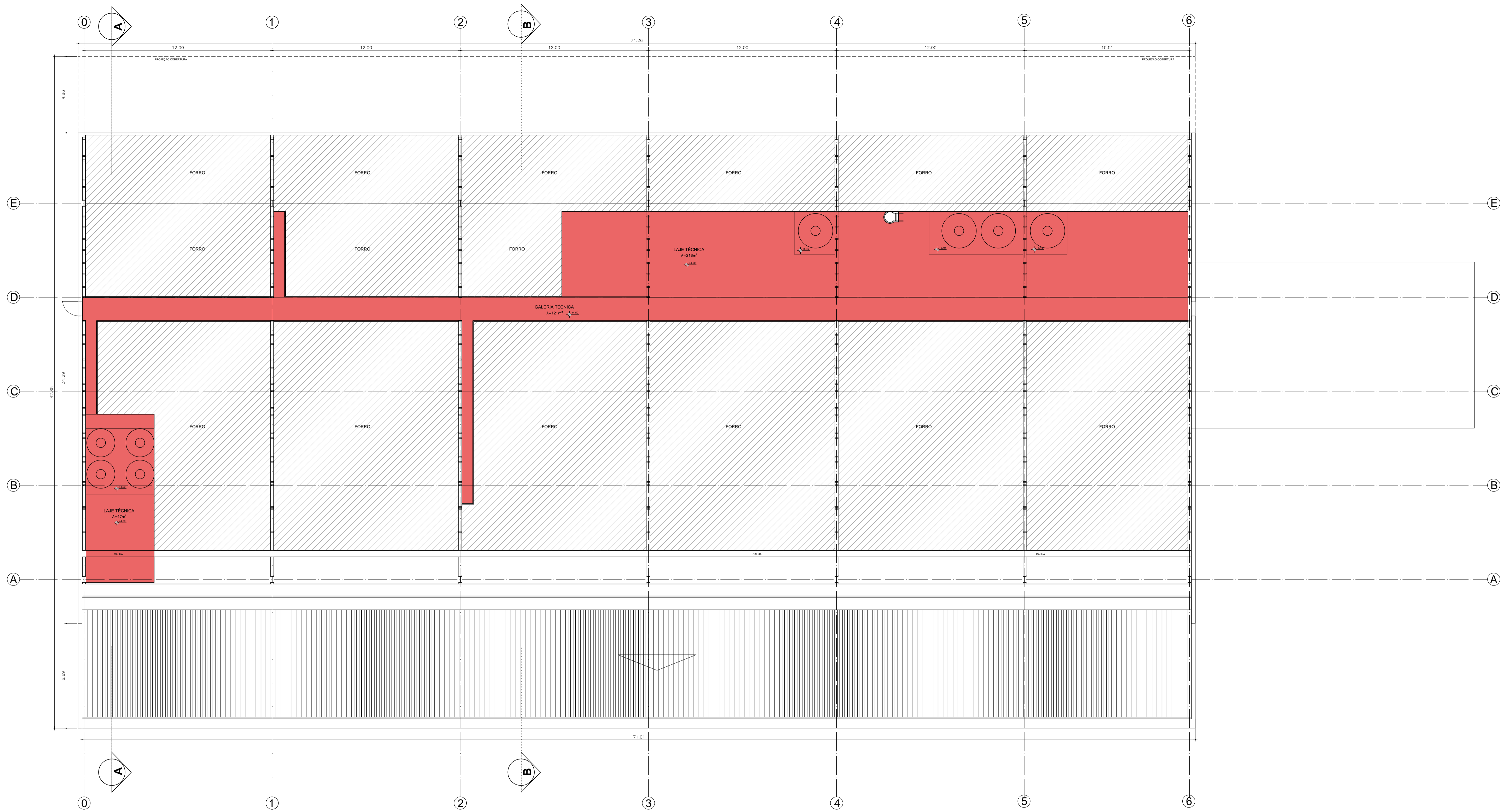
PLANTA BAIXA - NÍVEL TÉCNICO ESC. 1/125
