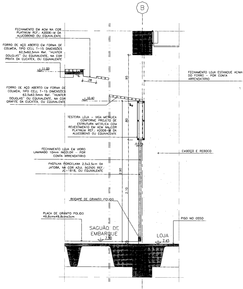
DETALHE 18 LOJAS EIXO "B - 06 E 12" - 1º PAVIMENTO (NÍVEL 7.50)
