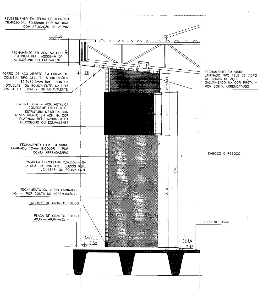
DETALHE 14 LOJAS EIXO "C - 05/06 E 12/13" - 1º PAVIMENTO (NÍVEL 7.50)
