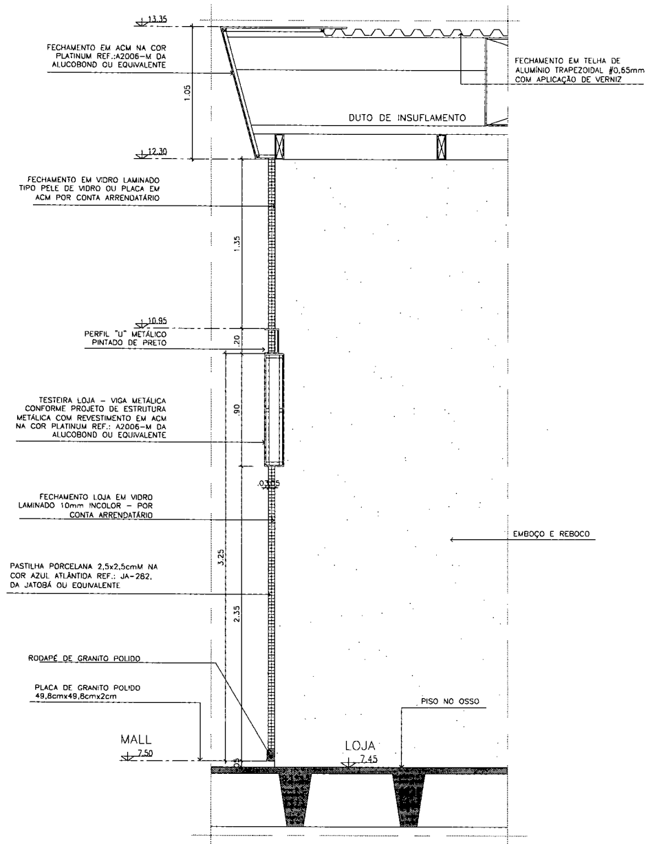
DETALHE 17 LOJAS EIXO "F / 01 A 06 - 12 A 17" - 1º PAVIMENTO (NÍVEL 7.50)
