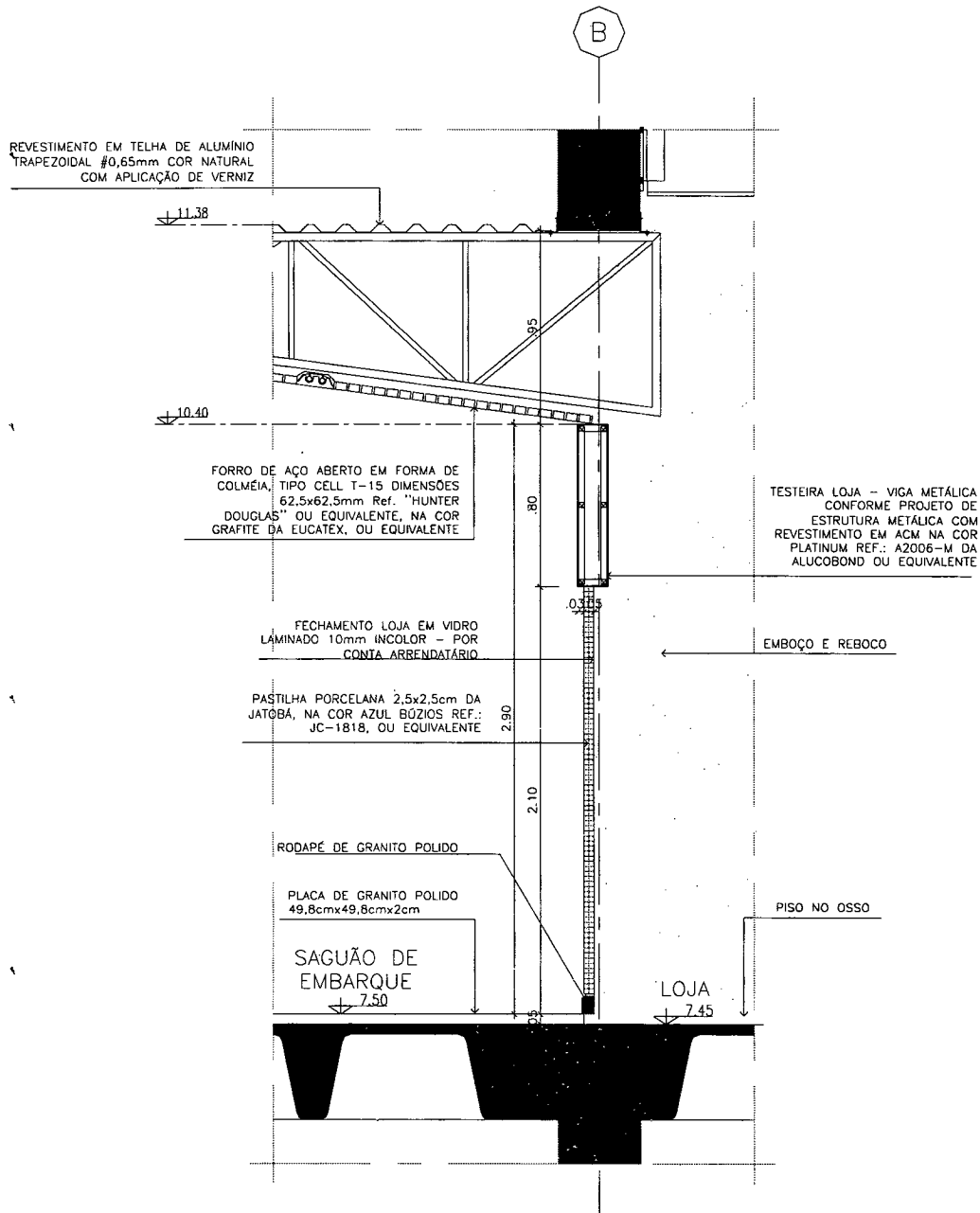
DETALHE 16 LOJAS EIXO "B - 01/06 E 12/16" - 1º PAVIMENTO (NÍVEL 7.50)
