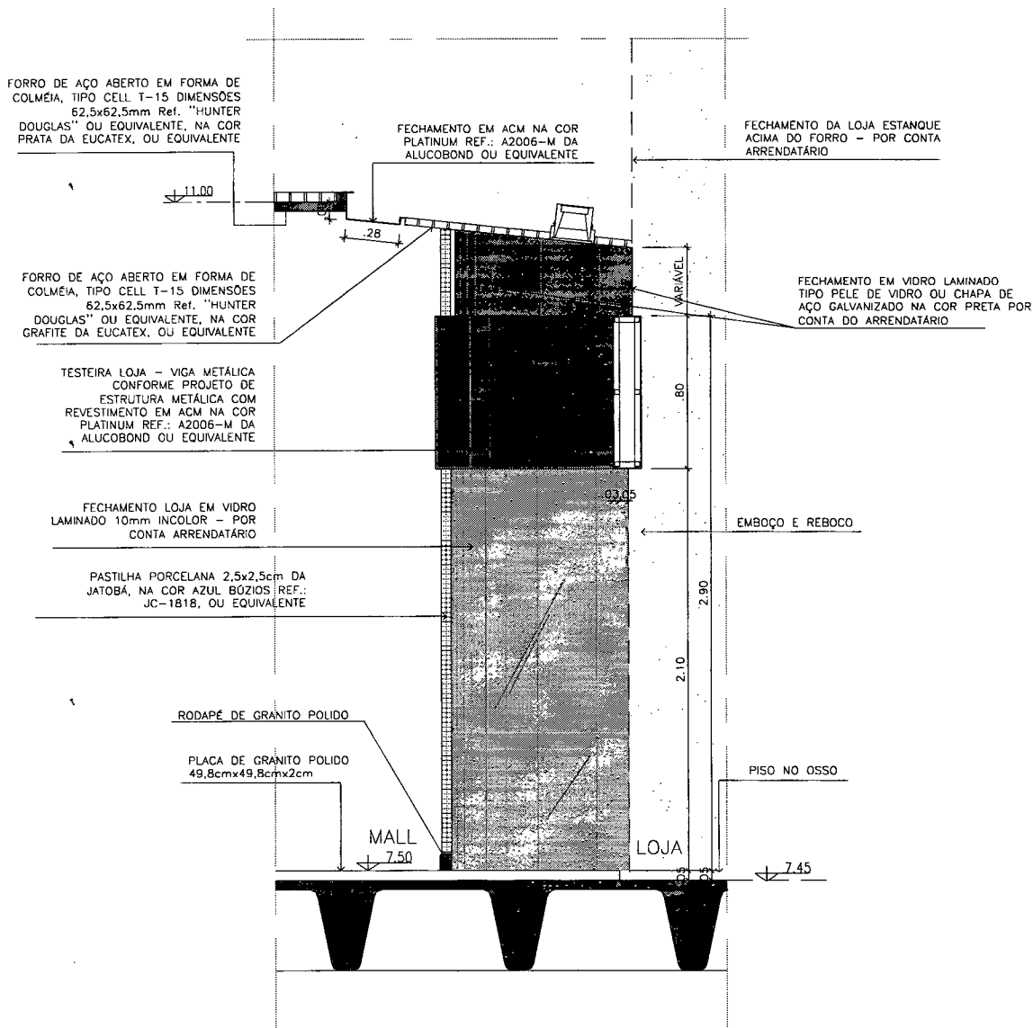
DETALHE 15 LOJAS EIXO "C - 06 E 12" - 1º PAVIMENTO (NÍVEL 7.50)
