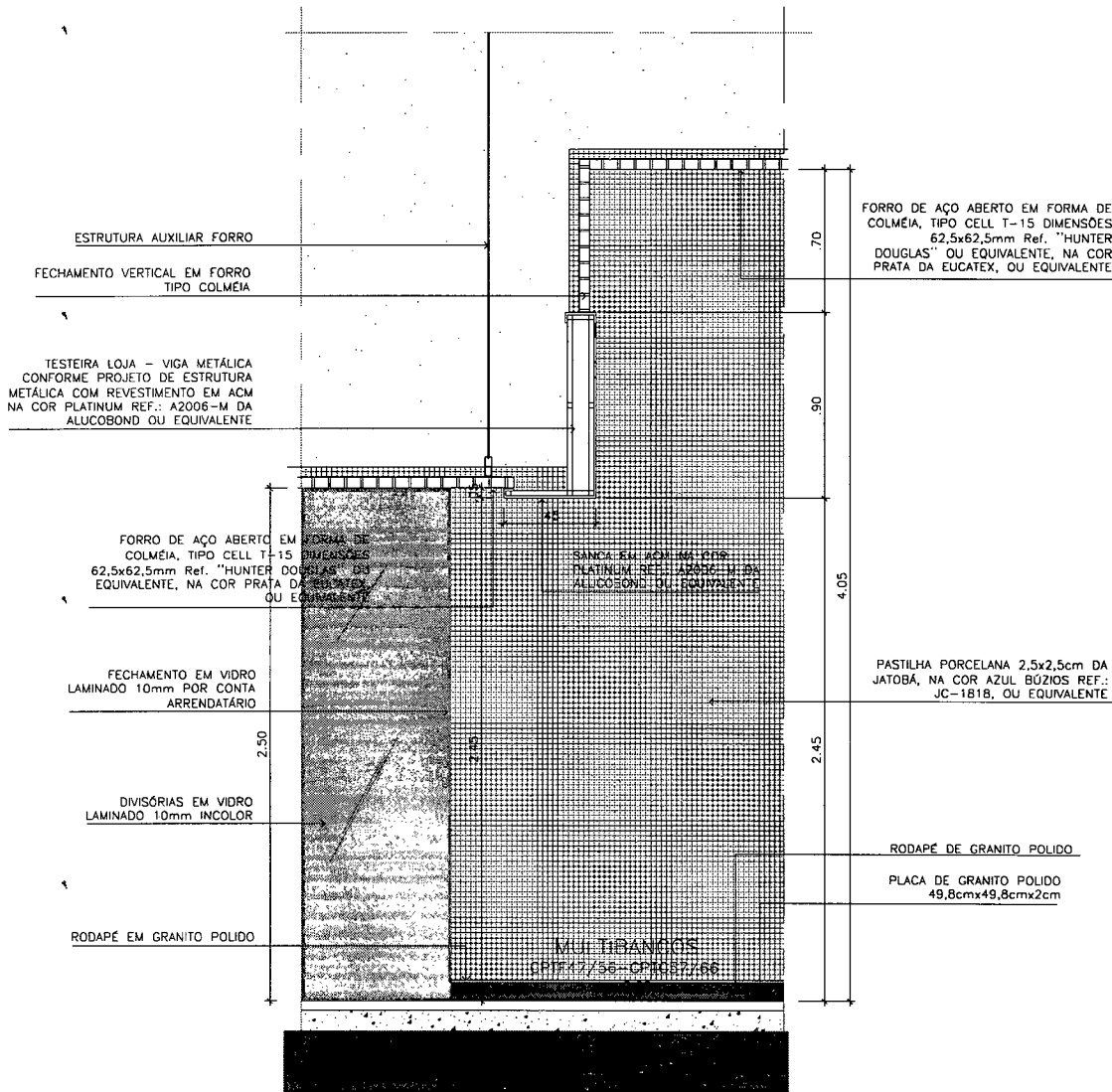
DETLAHE 11 MULTIBANCOS - EIXO "F" - PAV. TÉRREO (NÍVEL 0.00) ESCALA: 1/25
