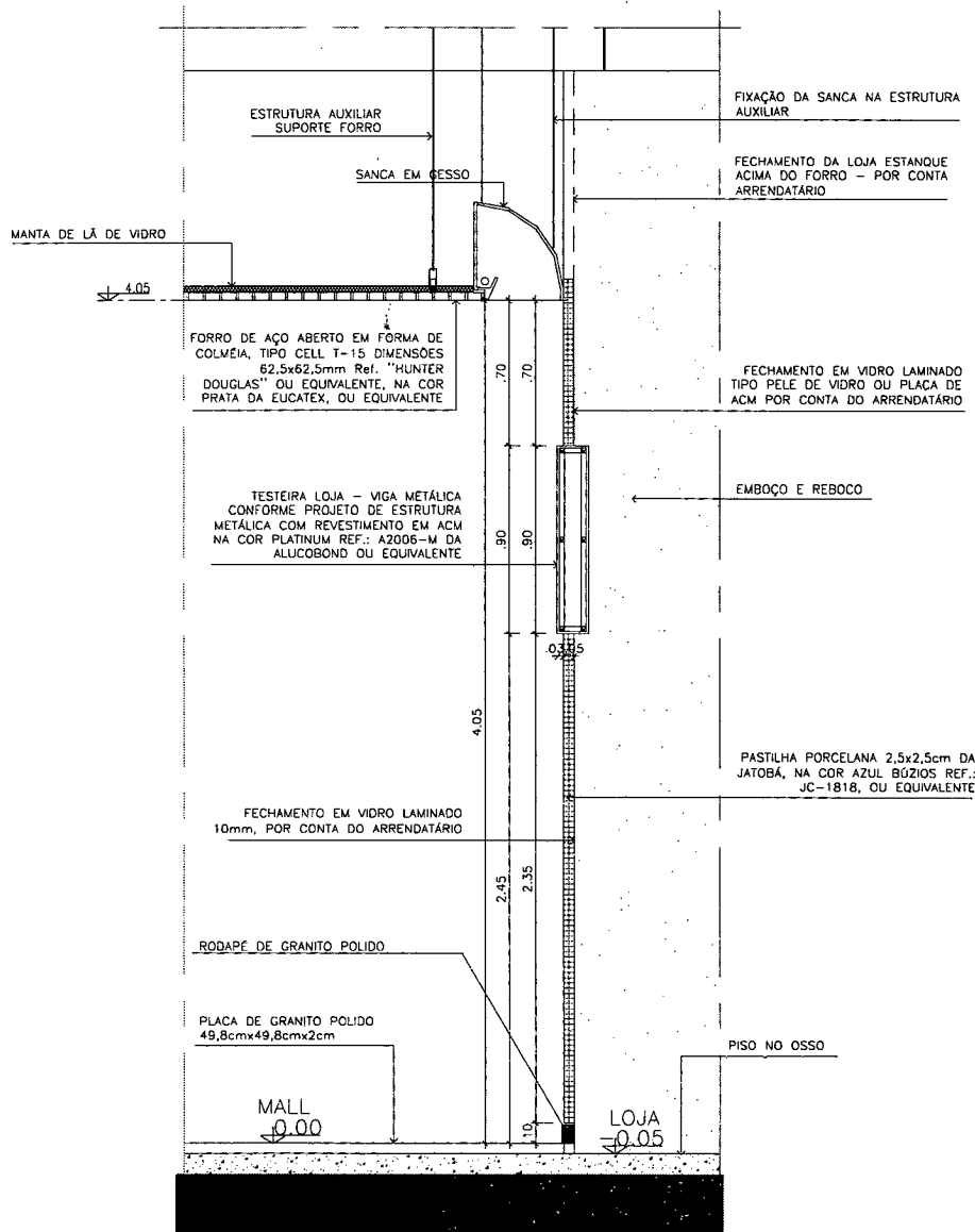
DETLAHE 09 LOJAS EIXO "F" - PAV. TÉRREO (NÍVEL 0.00)
