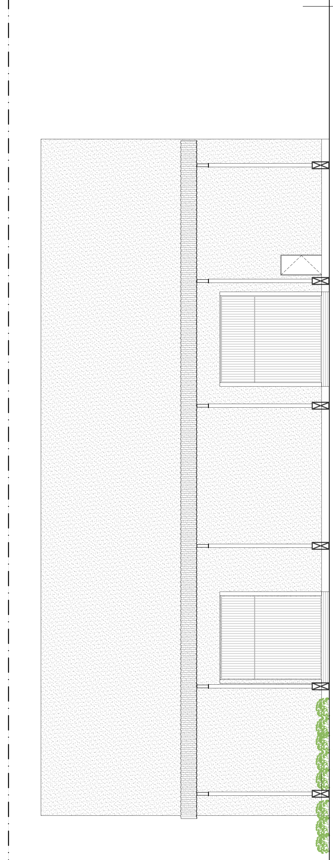
FACHADA NOROESTE TECA I - INFRAERO 1/100
