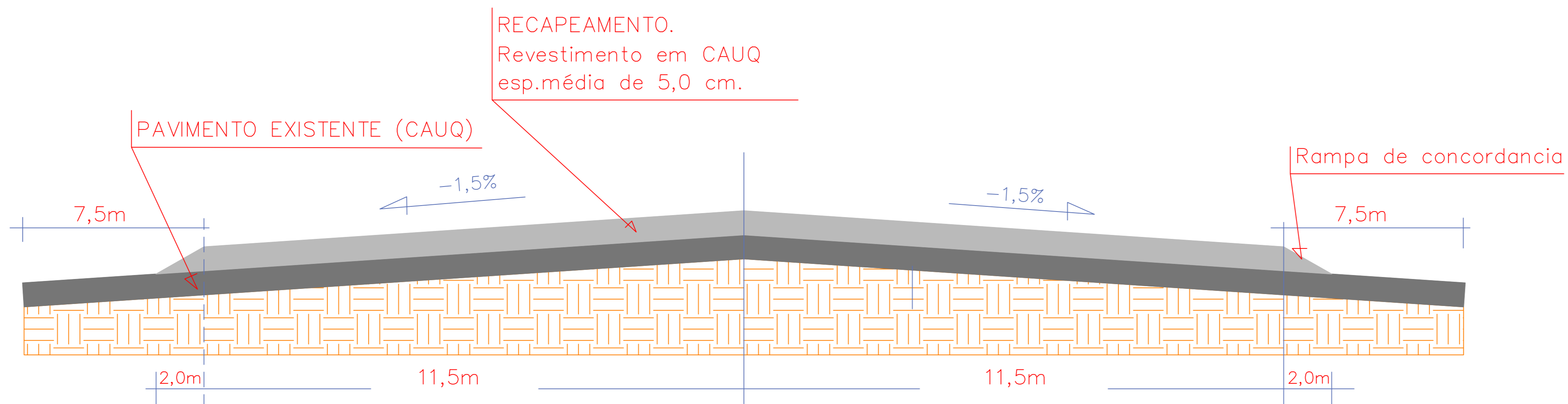
SEÇÃO TÍPICA ROLAMENTO (TÁXI) SEM ESCALA
