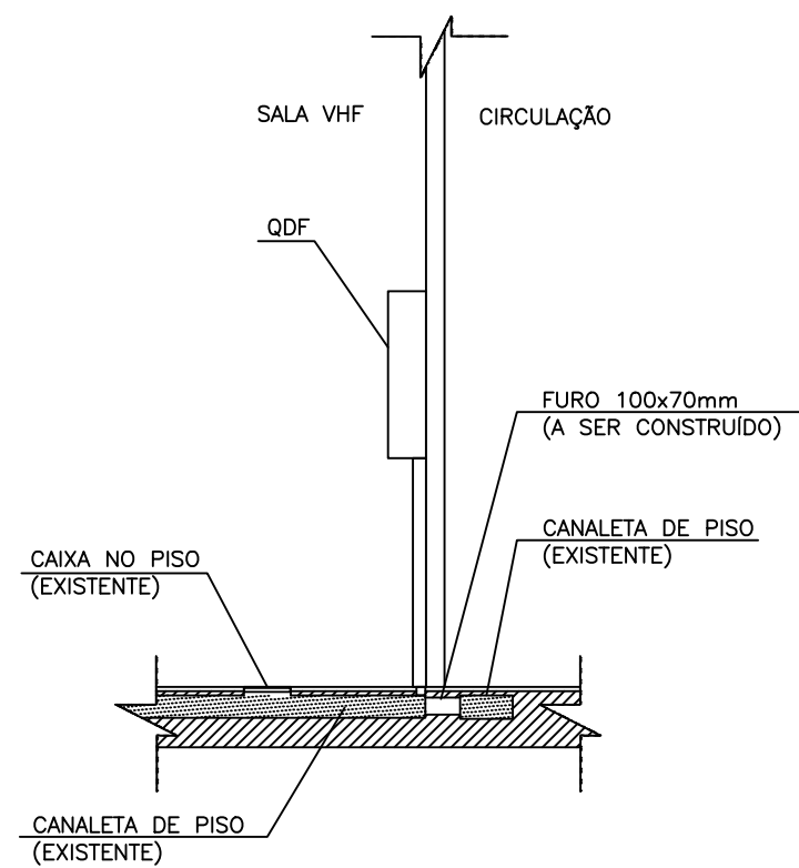
CORTE AA S/ ESC.
