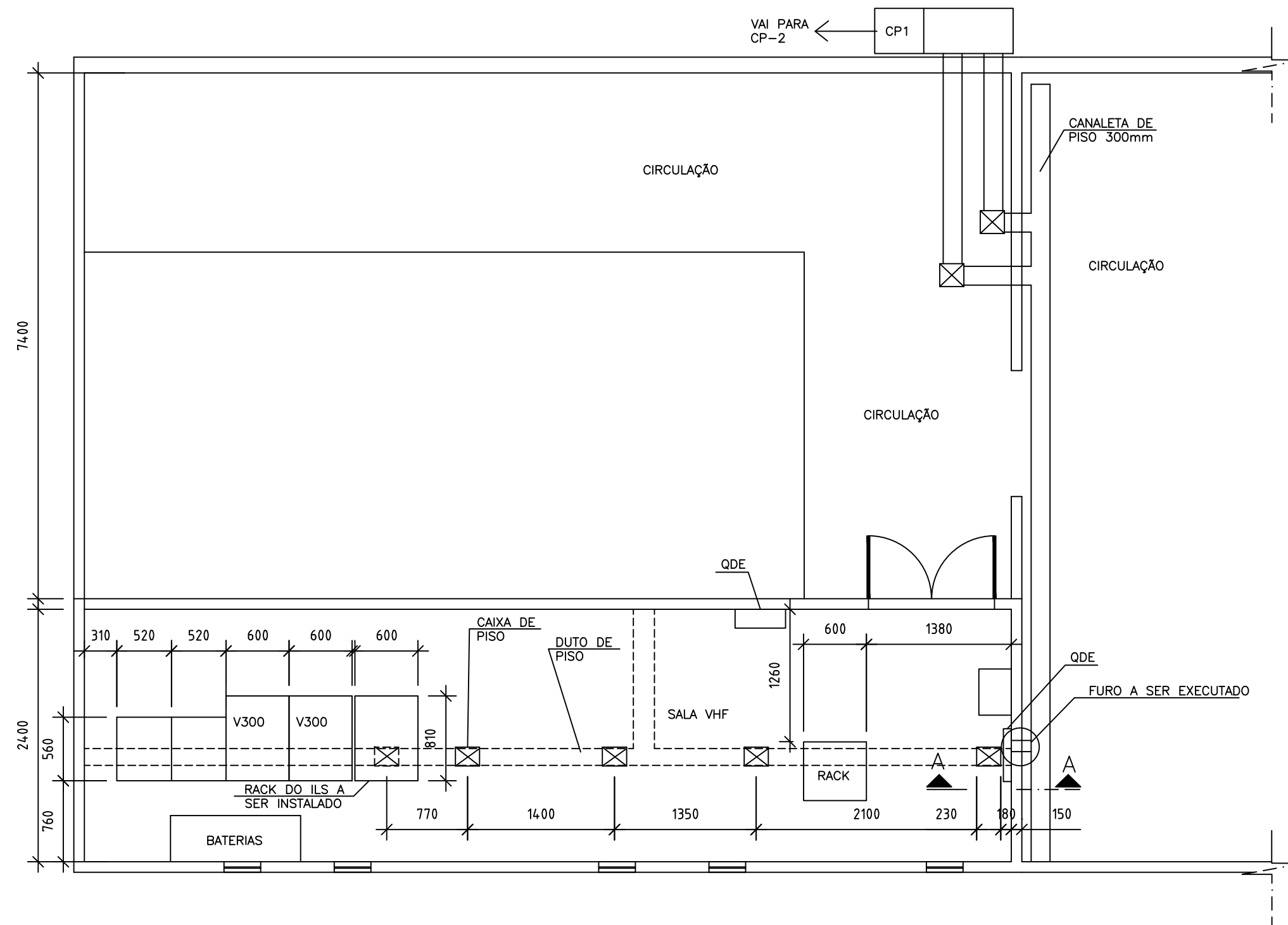
PLANTA BAIXA S/ ESC.
