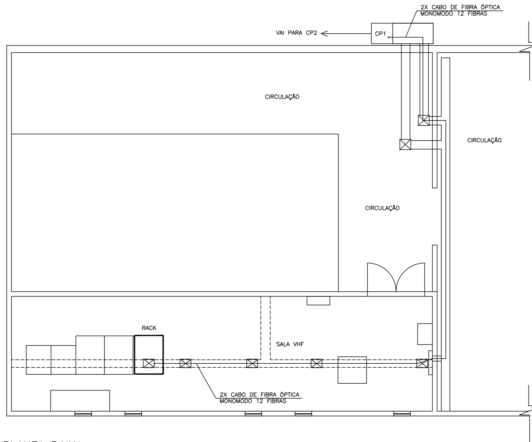
PLANTA BAIXA S/ ESC.
