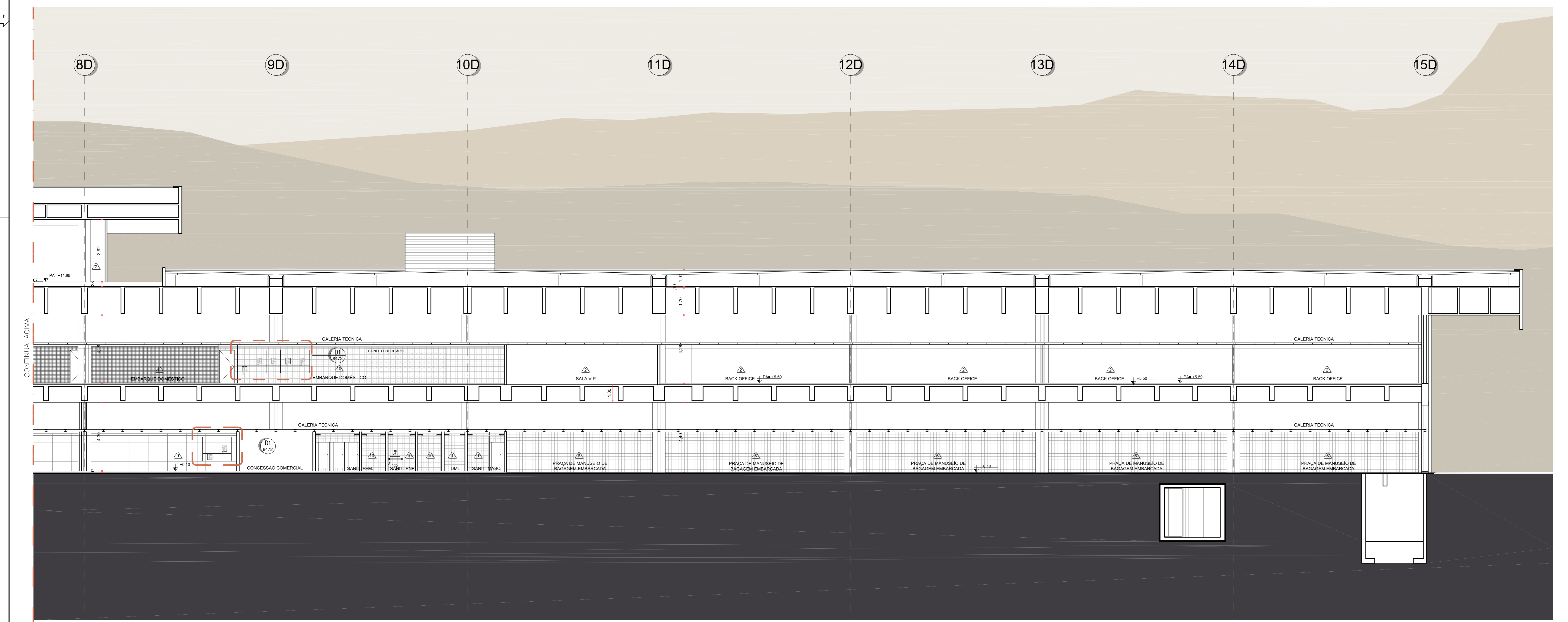
1 CORTE EE ESC: 1:100
